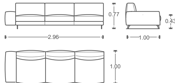
ELEMENTO CENTRAL CON BRAZO DER / IZQ 296 CM DE LARGO
