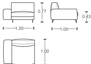
ELEMENTO CENTRAL CON BRAZO 120 CM DE LARGO
