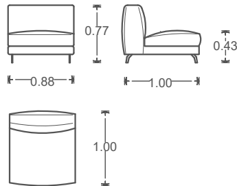
ELEMENTO CENTRAL SIN BRAZO 88 CM DE LARGO
